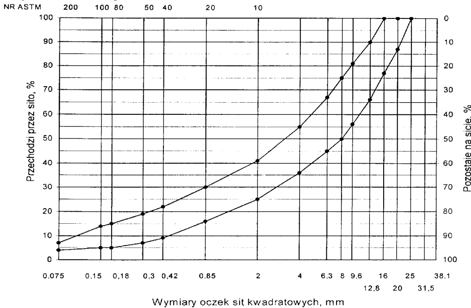
Rys. 2. Krzywe graniczne uziarnienia mieszanki mineralnej BA od 0 do 20 mm do warstwy wiążącej i wiążąco-wyrównawczej nawierzchni drogi o obciążeniu ruchem od KR3 do KR6
