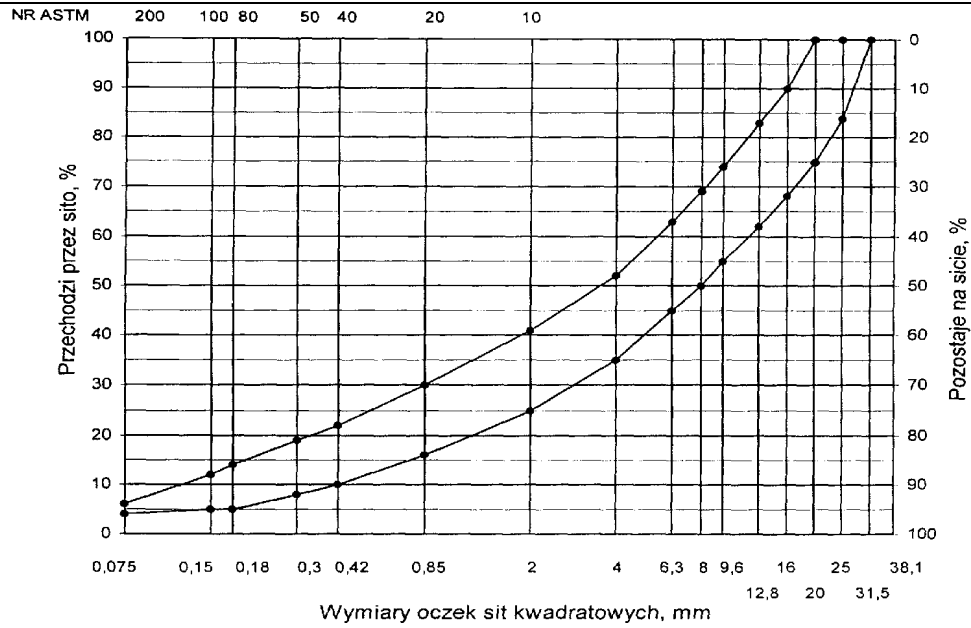
Rys. 1. Krzywe graniczne uziarnienia mieszanki mineralnej BA od 0 do 25 mm do warstwy wiążącej i wiążąco-wyrównawczej nawierzchni drogi o obciążeniu ruchem od KR3 do KR6
