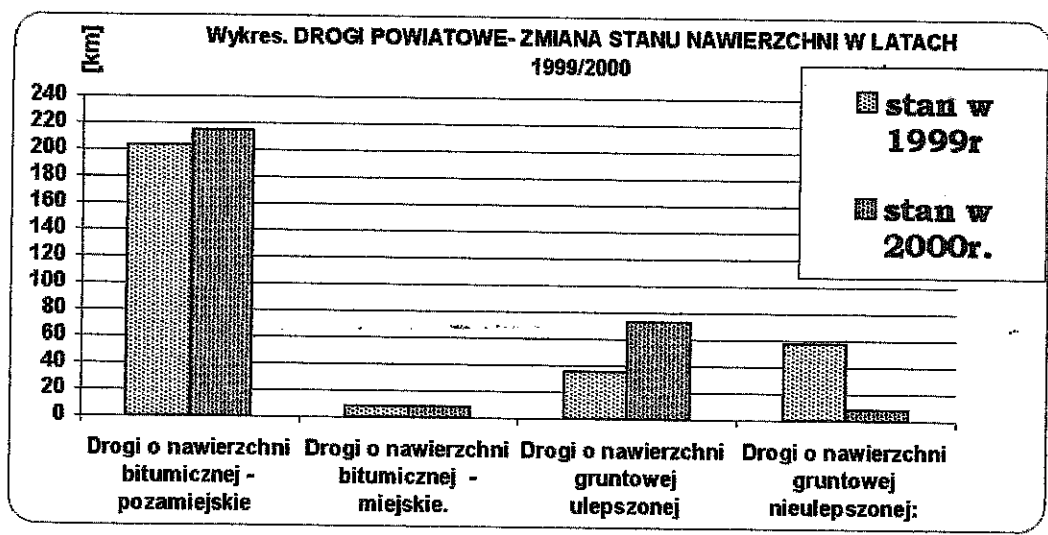
RYSUNEK NR ZMIAN STANU NAWIERZCHNI DRÓG POWIATOWYCH W LATACH 1999-2000
