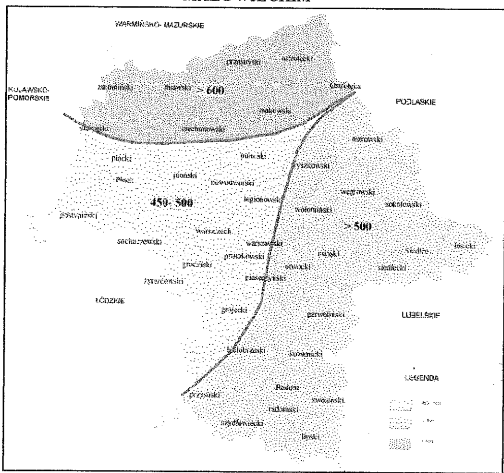
Rys. 5 ŚREDNIE ROCZNE OPADY (MM/ROK) W WOJEWÓDZTWIE MAZOWIECKIM
